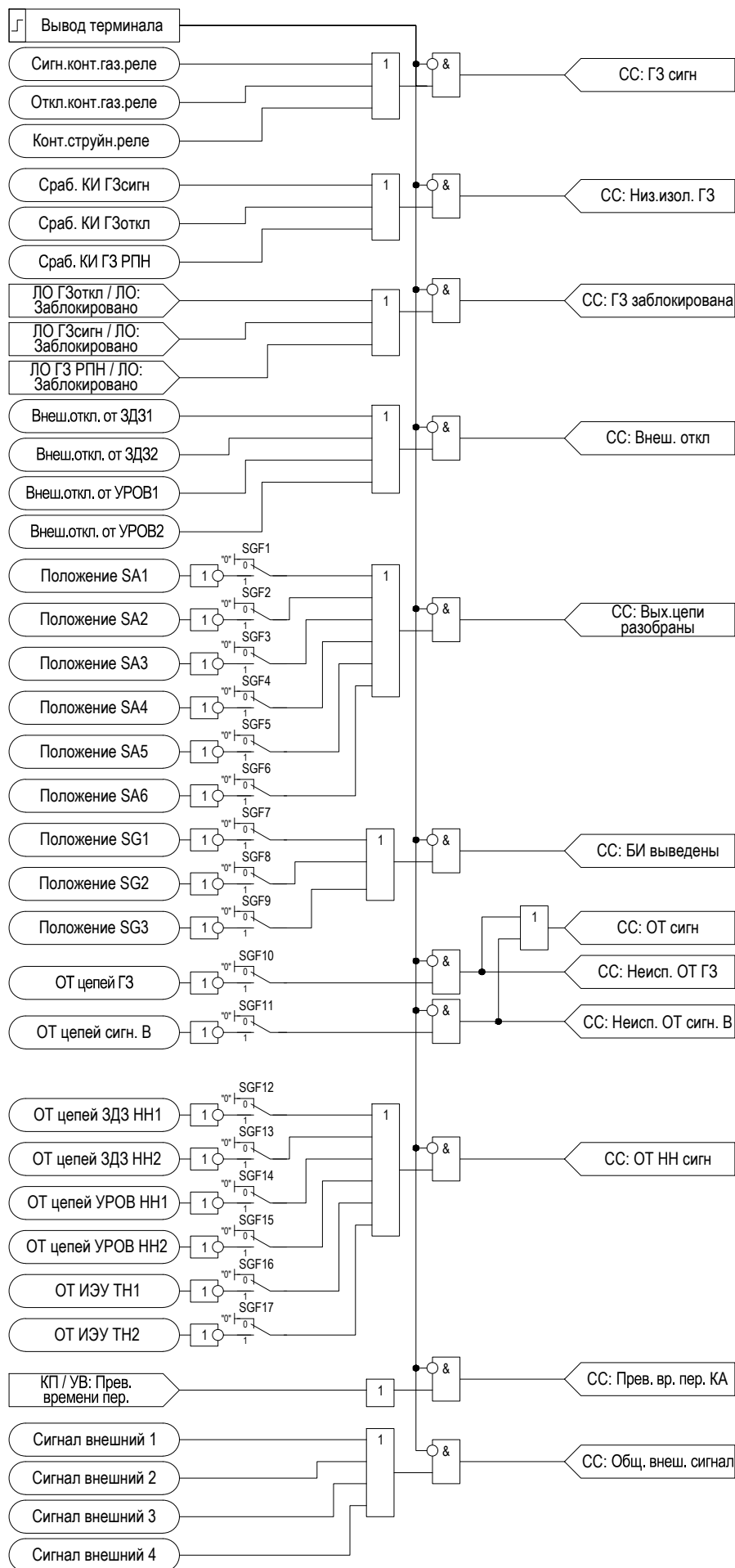
Рисунок 2.28 – Функциональная схема сборки сигналов
